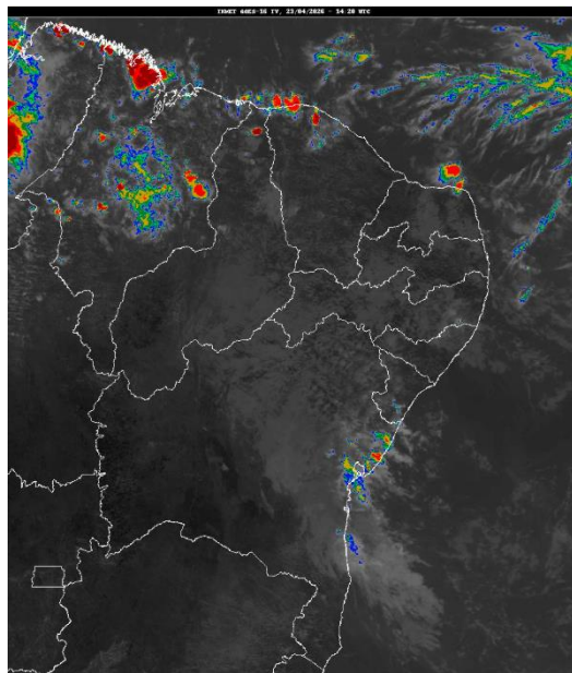
Figura 1 – Topo das nuvens (T°C).
