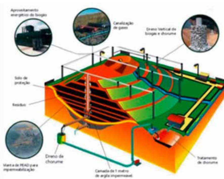
Figura 156: Ilustração de um aterro sanitário.
