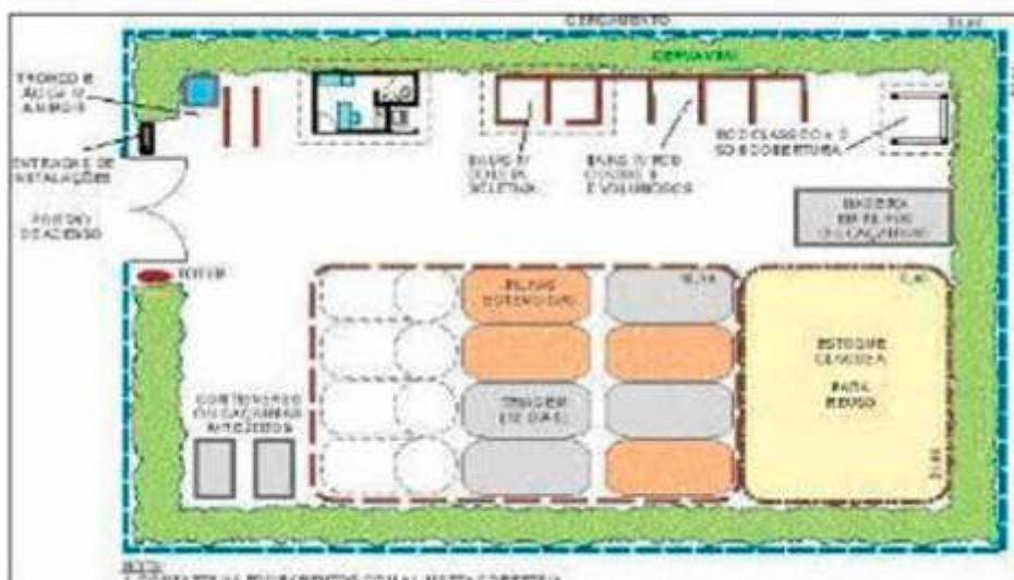
Figura 149: Layout típico para PEV Central Simplificado.
