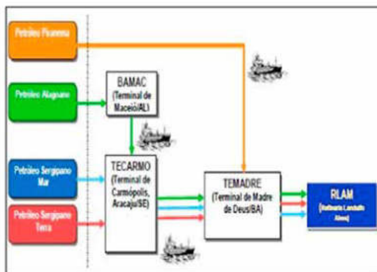
Figura 143: Fluxograma do Petróleo da UN-SEAL. Fonte: Petrobras – UN-SEAL, 2010 apud Sergipe, 2009.
